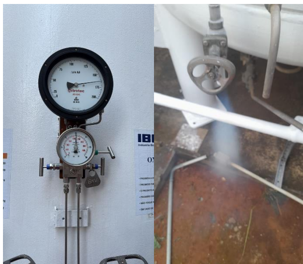
Monitoramento da pressão interna do tanque e alívio de pressão.
